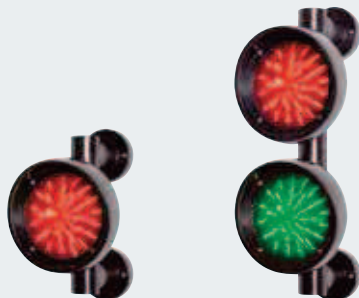
Signalno svetlo Ø 150 mm Crveno, u plastičnom kućištu sa držačem, IP 65
