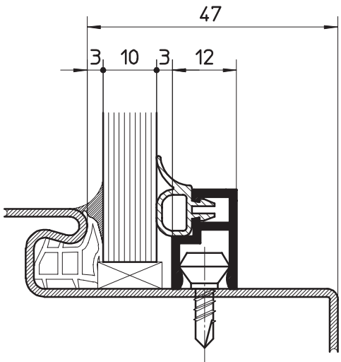
Glasdicke 24 mm
