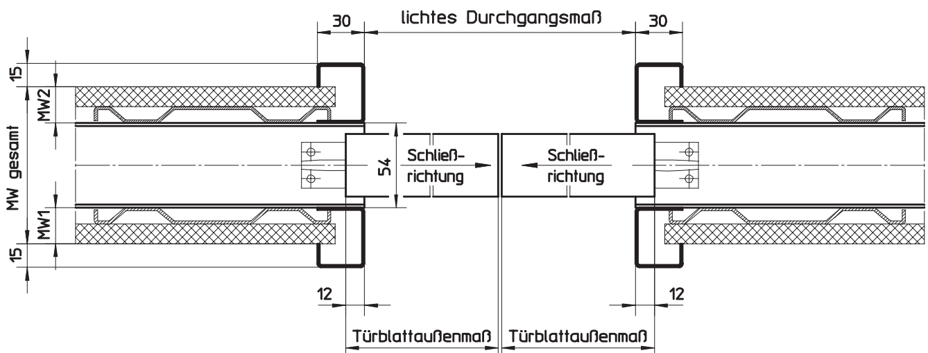
Schnitt B-B
