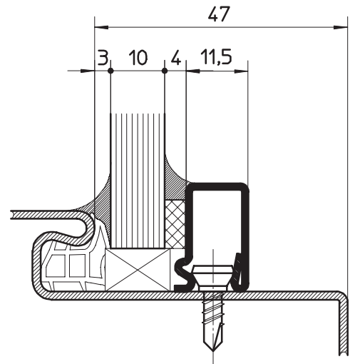
Glasdicke 24 mm
