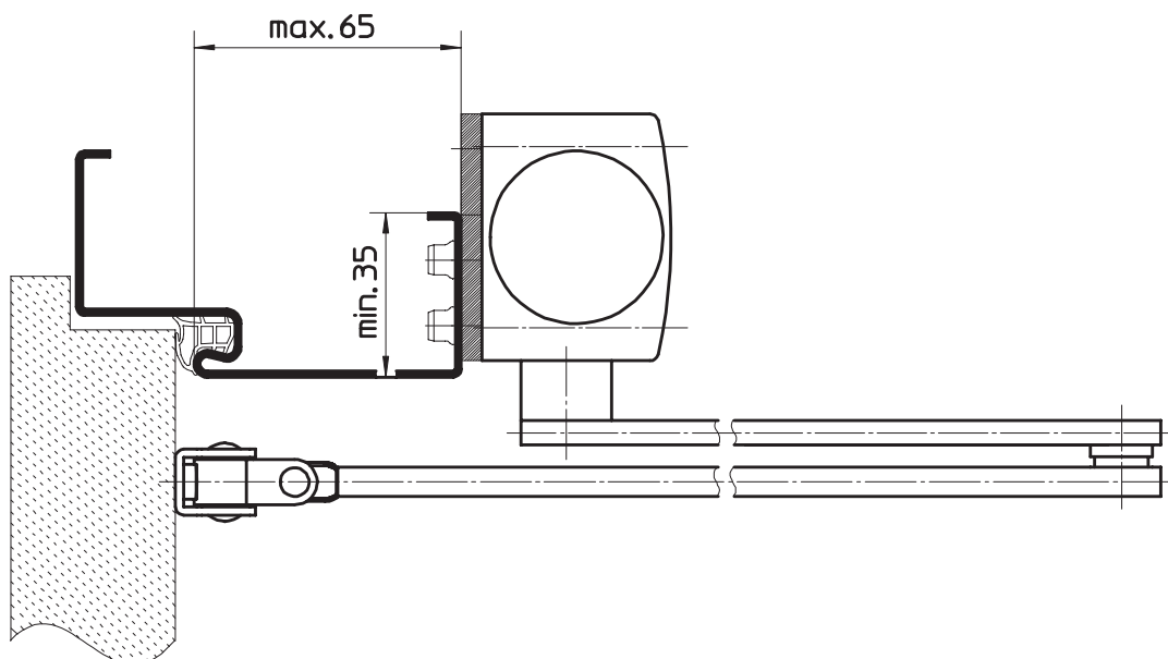
gegenbandseitige Normalmontage
