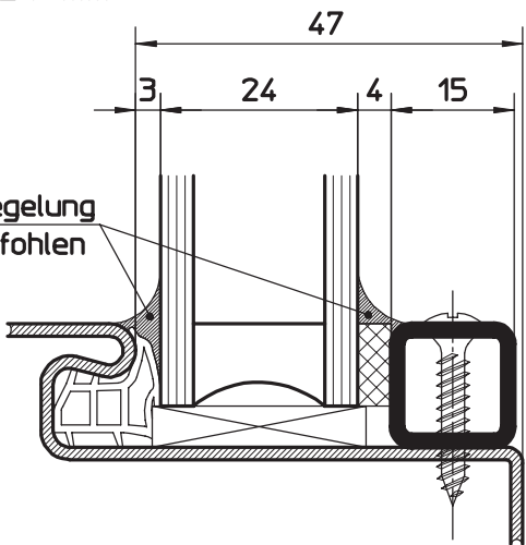
Glasdicke 24 mm
