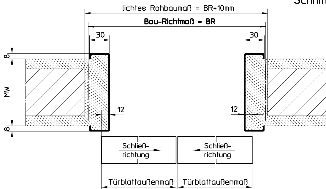
Schnitt B-B
