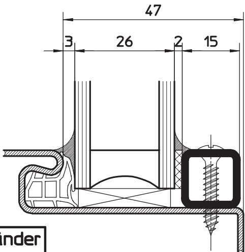
Glasdicke 26 mm
