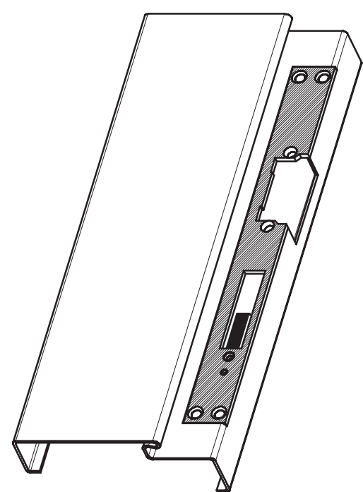
gefälzte Ausführung
