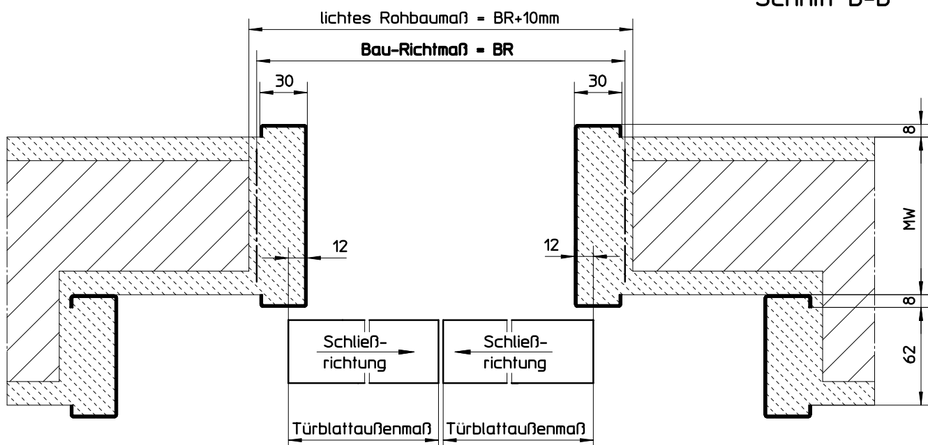
Schnitt B-B
