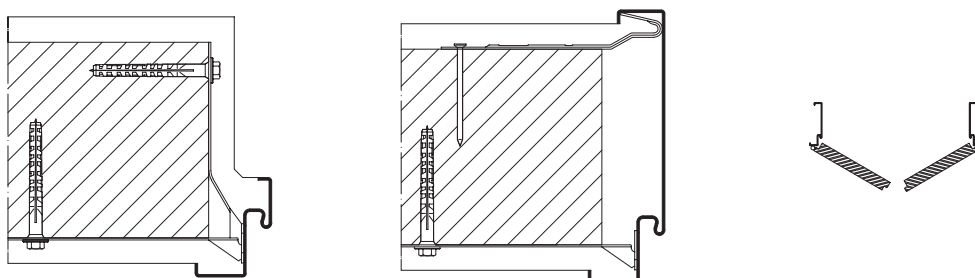
Maße für 2-flügelige Ausführung
