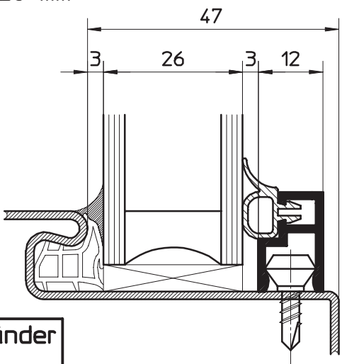
Glasdicke 26 mm
