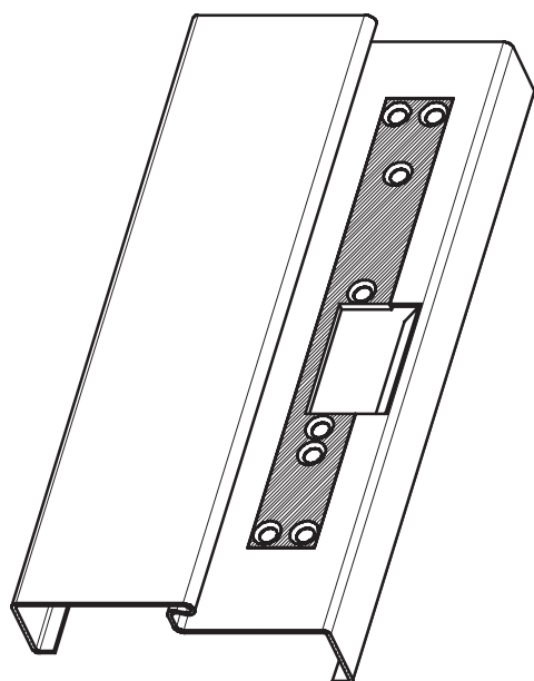
ungefälzte Ausführung
