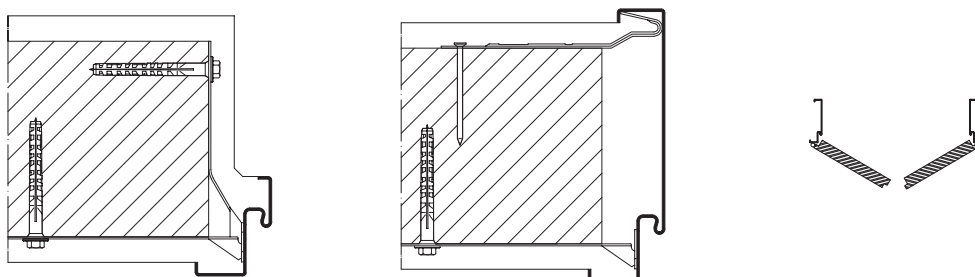
Maße für 2-flügelige Ausführung Ganzglastürblätter
