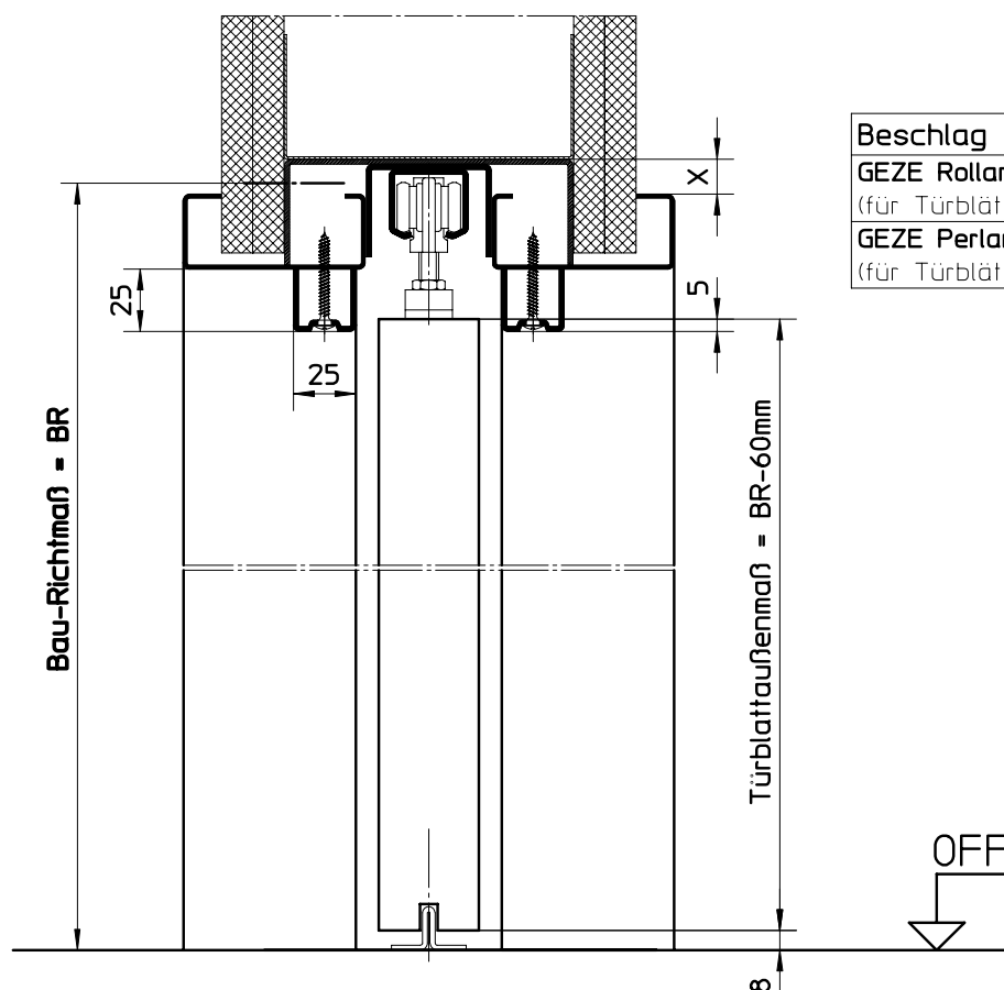
Schnitt A-A
