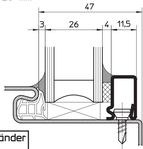
Glasdicke 26 mm
