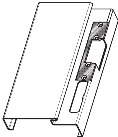
gefälzte Ausführung
