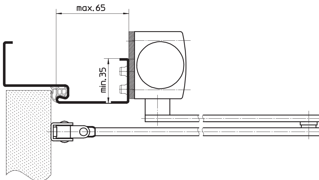
gegenbandseitige Normalmontage
