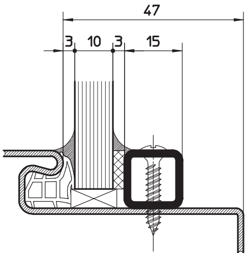
Glasdicke 10 mm
