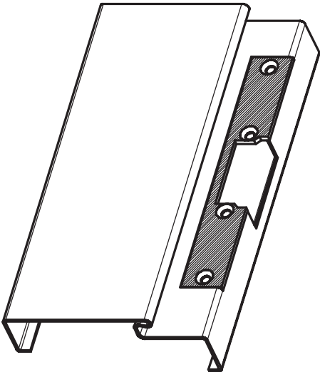
gefälzte Ausführung
