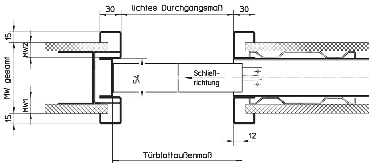
Schnitt B-B
