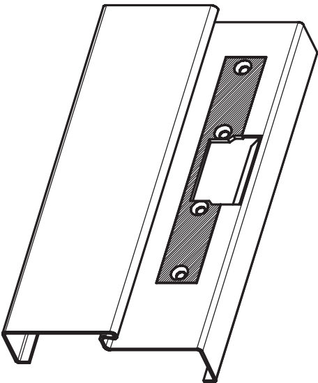
ungefälzte Ausführung
