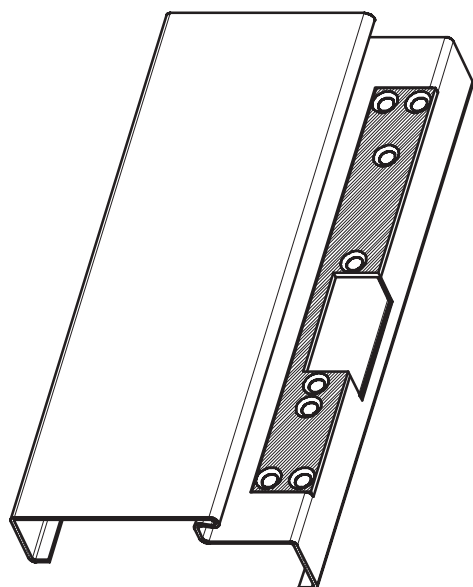
gefälzte Ausführung
