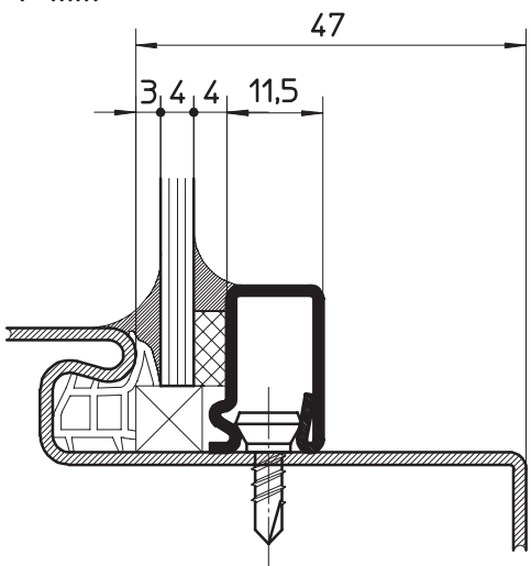
Glasdicke 6 mm
