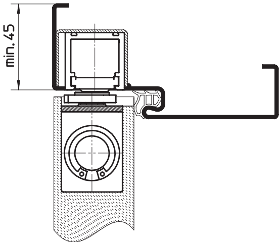
Türschließer Gr.2-4 mit E-Gleitschiene
