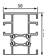
Profil za proširenje 50 mm
