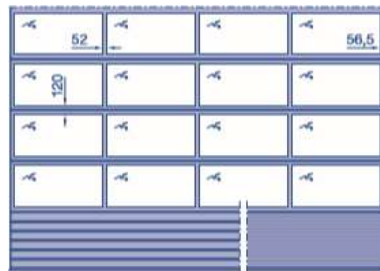
Osnovni model (bez pešačkih vrata) sa ravnomernom podelom polja u širini
