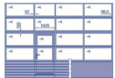
Model sa pešačkim vratima i prag
