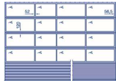
Osnovni model (bez pešačkih vrata) podela polja po širini istog izgleda kao pešačka vrata
