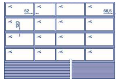
Osnovni model (bez pešačkih vrata) podela polja po širini istog izgleda kao pešačka vrata
