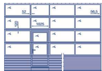
Model sa pešačkim vratima i prag
