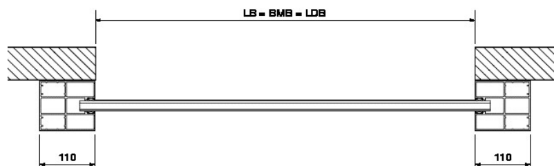
Montaža ispred ili iza otvora
