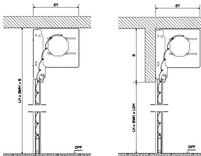
Montaža u otvor
