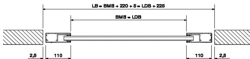
Montaža u otvor
